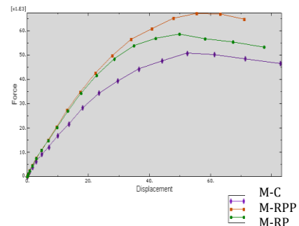
Figure 4 : Comparaison des courbes de capacités.
