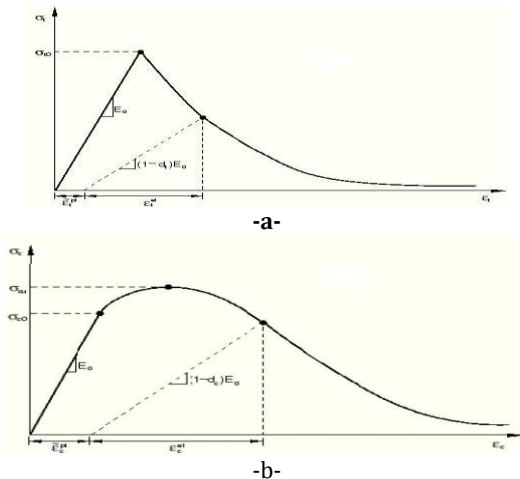
Figure 1 : comportement uni axial du béton a : traction b:compression. [9]
