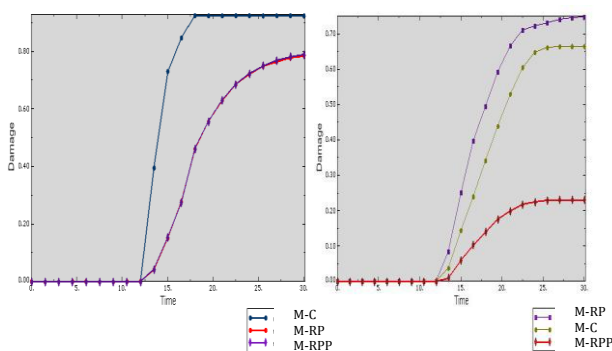
Figure 6 : comparaison des dommages en traction dans un élément de béton.
