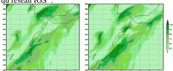
FIGURE 2 – L'humidité relative à 700hPa prévue pour le 21 Septembre à 6h pour EXP-ref (à gauche) et EXP-gps (à droite).
