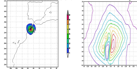
FIGURE 1 – Incrément d'analyse de l'humidité relative pour EXP-1obs au niveau 700hpa (à gauche) et coupe longitudinale verticale de cet incrément (à droite).
